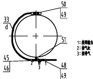
平台制动手接管示意图
