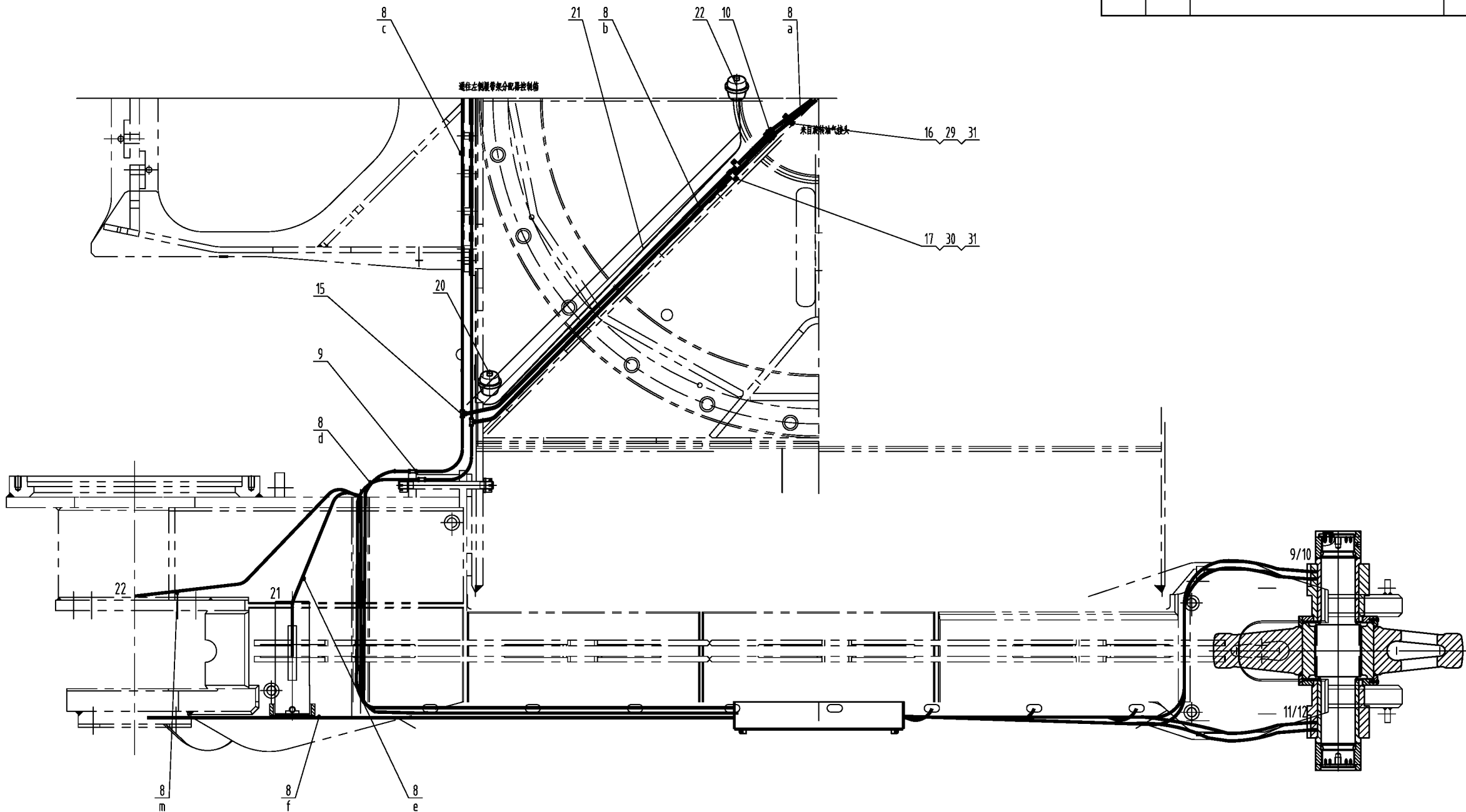
分配器盒内件热带布置图 1:5
