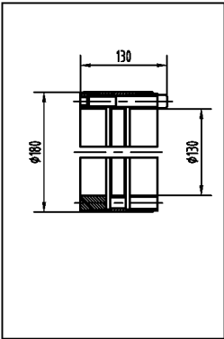
胀紧套放大图
