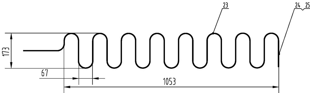
分配器盒内件热带布置图 1:5
